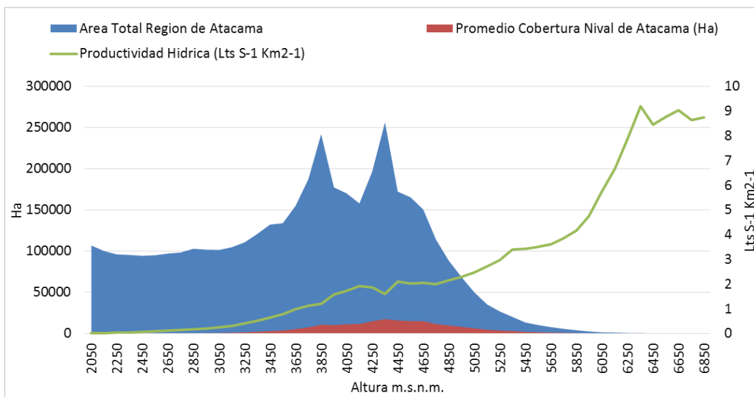
Figura 17: Área total de la Región de Atacama, y la cobertura nival promedio en todas las imágenes analizadas en la región, así como su porcentaje en base al área total.
