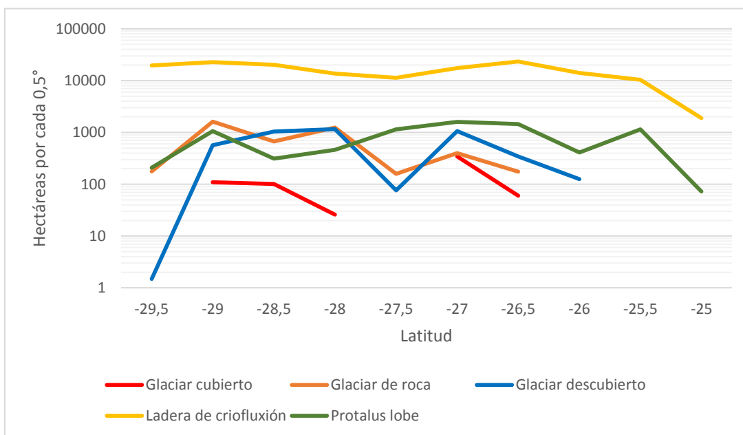
Figura 5: Distribución latitudinal del área de crioformas en la región de Atacama.
