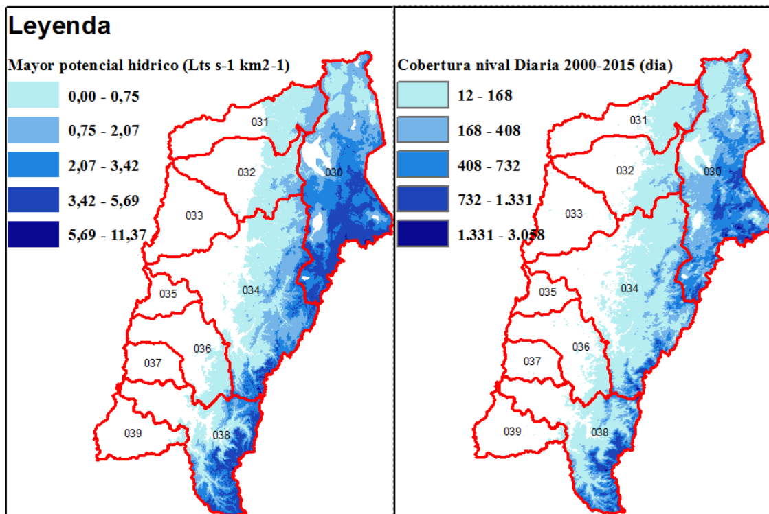
Figura 12: A la izquierda, Subcuencas con mayor productividad hídrica promedio, y a la derecha cobertura nival diaria. (José Espinoza)
