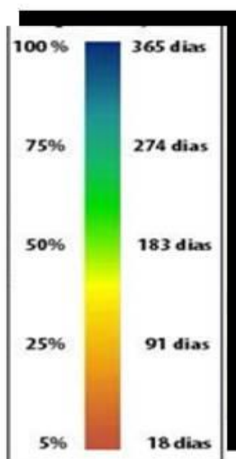
Figura 18: mapeo diario de nieve estacional: Los colores verdes a azul grafican las áreas con mayor cantidad de días con nieve.
