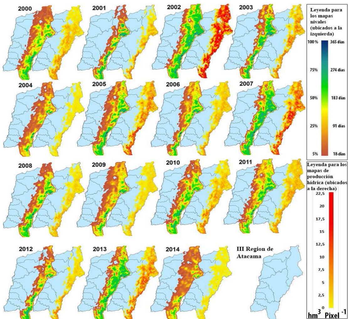
Figura 15: Mapas del manto nival (izquierda) y la de fusión de esté (derecha), para los años 2000 al 2014 (Figura 4.1.1, Espinoza, 2016)
