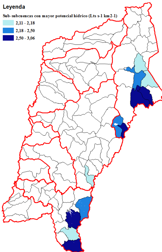
Figura 16: Sectorización de potencial hídrico presente en la Región de Atacama.
