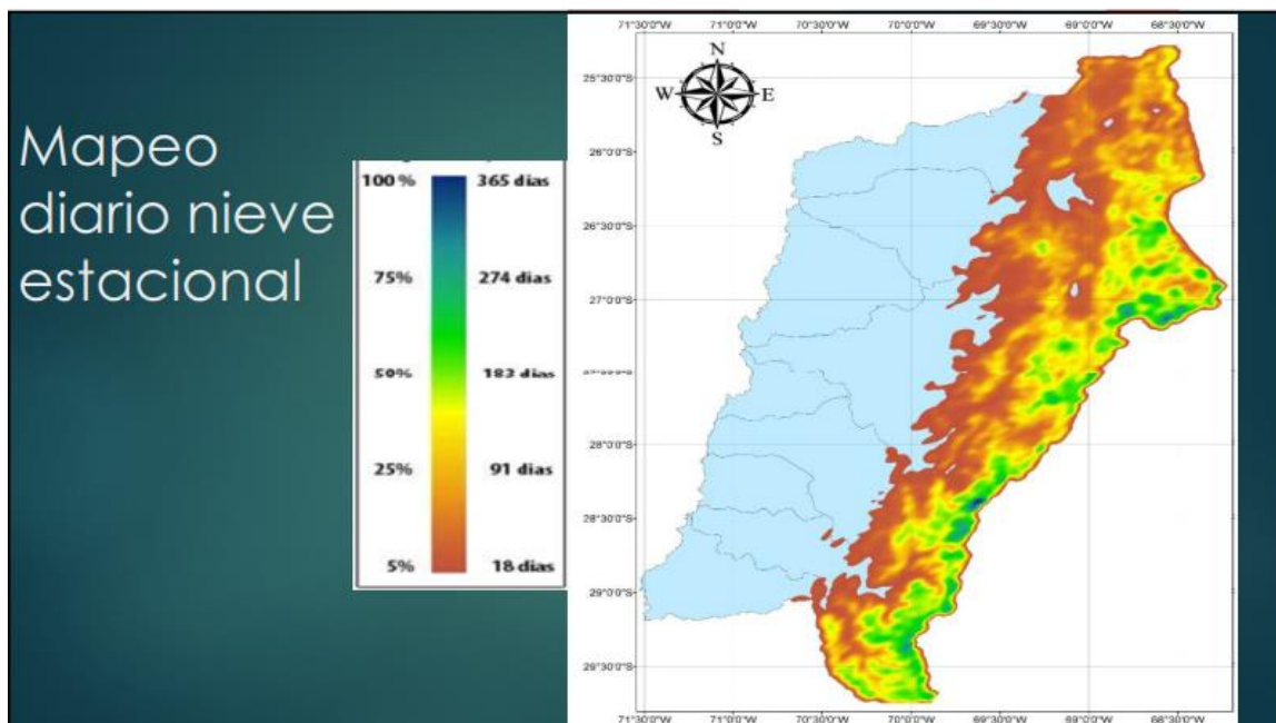
Figura 10: Mapeo diario nieve estacional: Cantidad de nieve presente estadísticamente en un sector.
