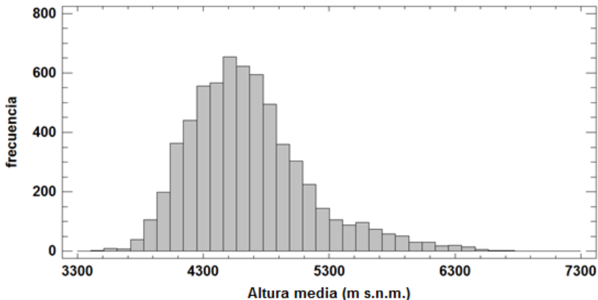
Figura 9: Histograma de frecuencia para altura media en m s.n.m., de los 6.280 cuerpos criosféricos relevados para la región de Atacama.
