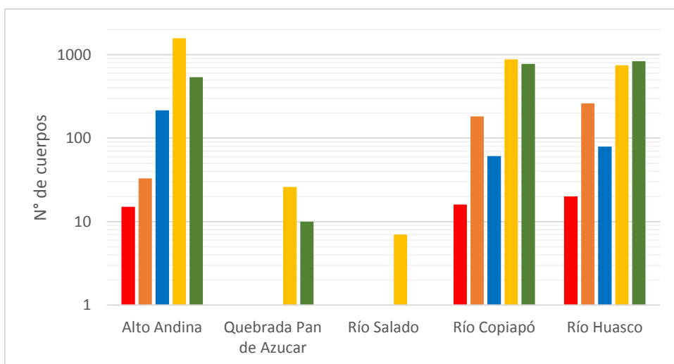
Figura 8: Cantidad de cuerpos de crioformas por cuencas principales de la región de Atacama (Código de color figura anterior). (4.1.)
