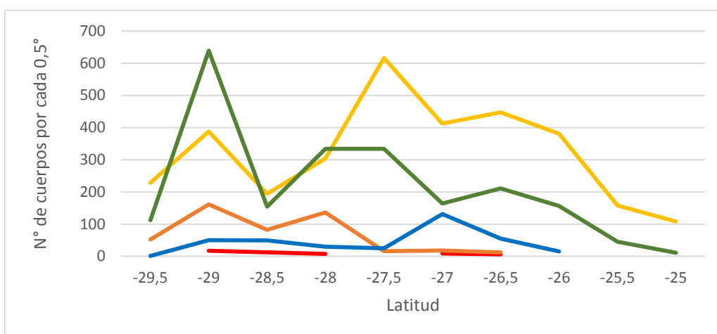
Figura 6. Variación latitudinal de la cantidad de cuerpos de crioformas por clase para la región de Atacama.
