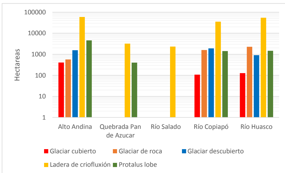
Figura 7: Distribución del área de crioformas por cuencas principales en la región de Atacama. (Elaboración propia).
