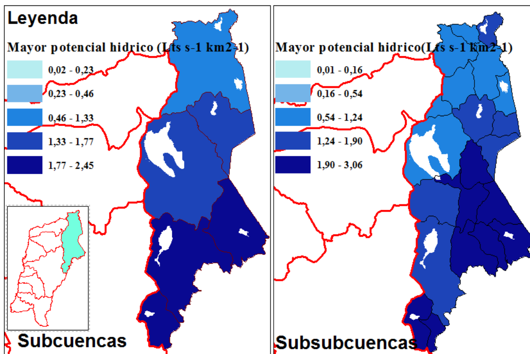
Figura 13: Productividad nival en diferentes cuencas y subcuencas de Atacama
