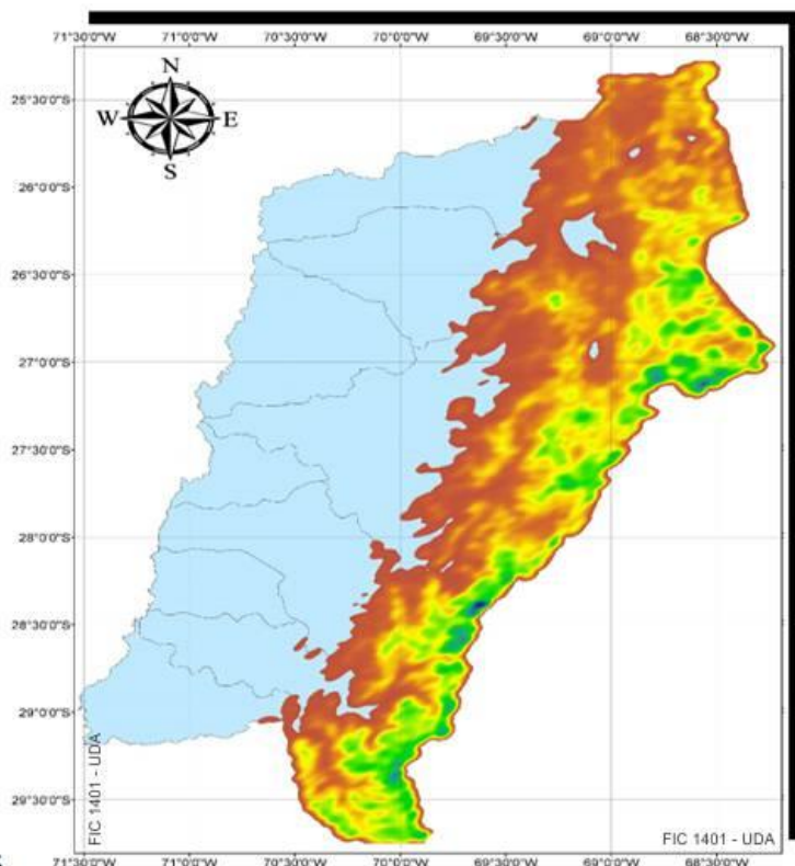
Figura 18: mapeo diario de nieve estacional: Los colores verdes a azul grafican las áreas con mayor cantidad de días con nieve.
