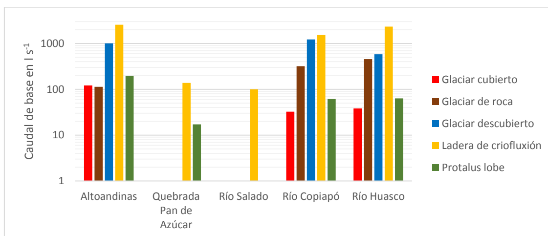
Fig. 11: Productividad hídrica en litros por segundo, por clase y por cuencas principales, eje y en escala logarítmica en base 10. (García, 2016)
